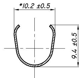
CORTE B-B
