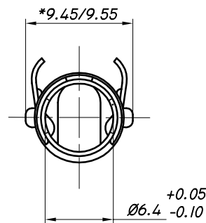
CORTE C-C
