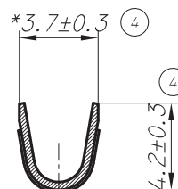
CORTE B-B
