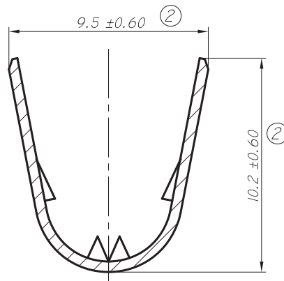
CORTE B-B
