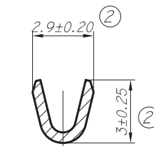
CORTE C-C
