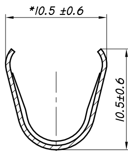
CORTE A-A
