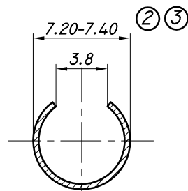
CORTE D-D
