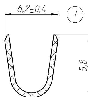
SECCIÓN L-L
