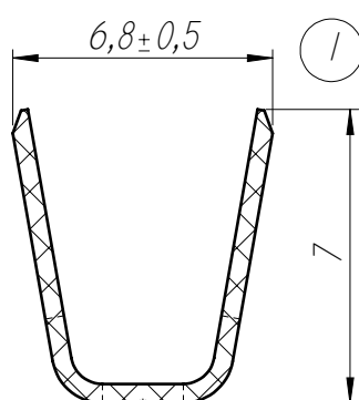
SECCIÓN J-J
